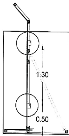
SECCIÓN
